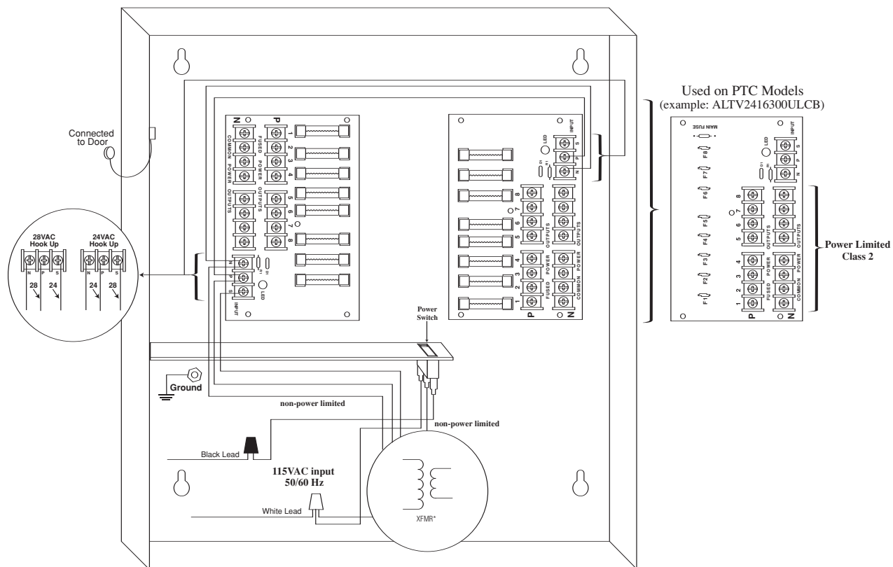
Fig. 2 ALTV2416300UL • ALTV2416300ULCB
