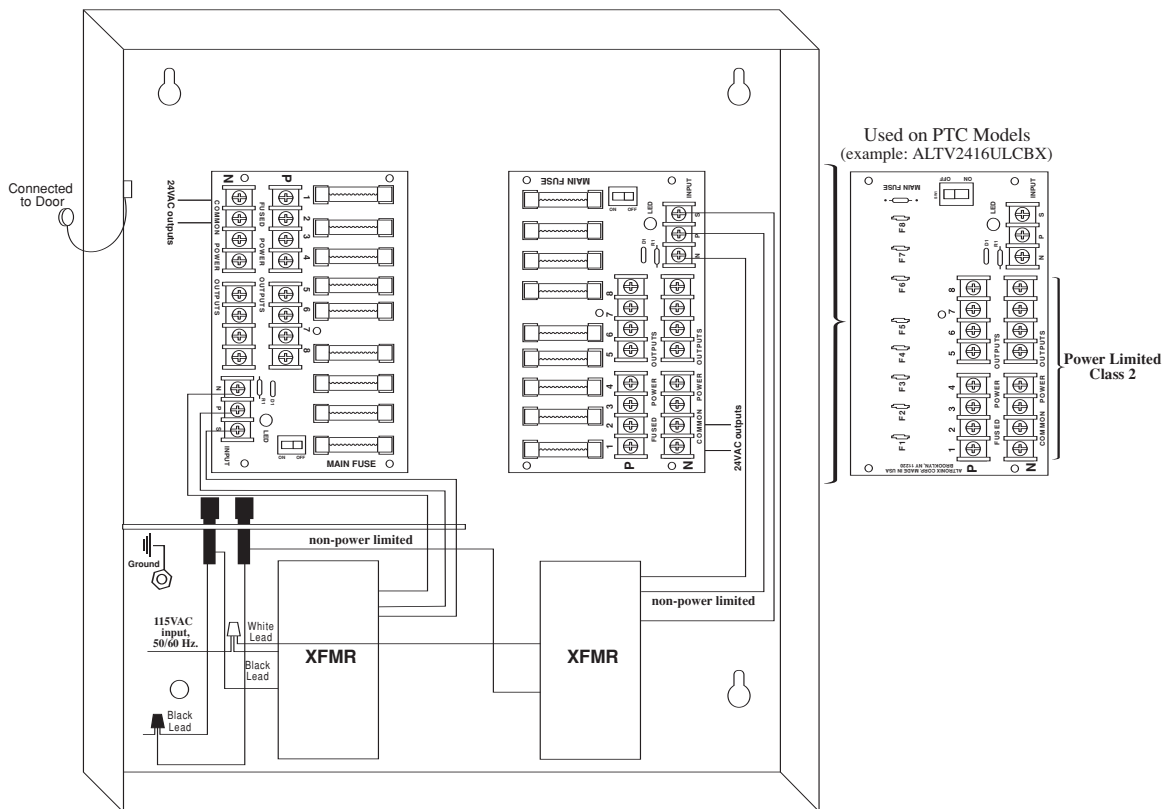
Fig. 2 ALTV2416300UL • ALTV2416300ULCB
