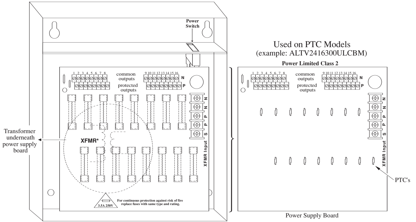
Fig. 3 ALTV2416300ULM • ALTV2416300ULCBM
