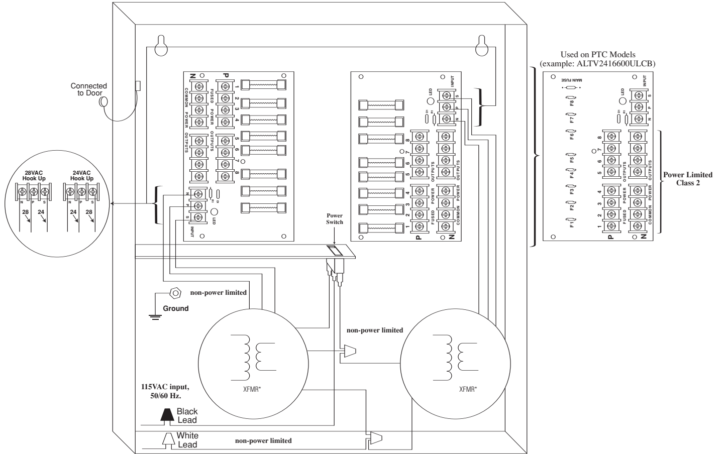
Fig. 4 ALTV2416600UL • ALTV2416600ULCB
